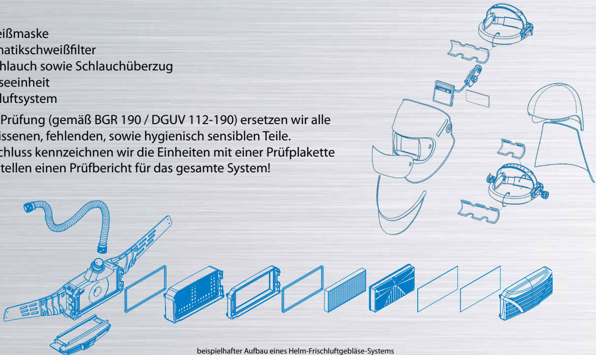
beispielhafter Aufbau eines Helm-Frischlufthebläse-Systems
